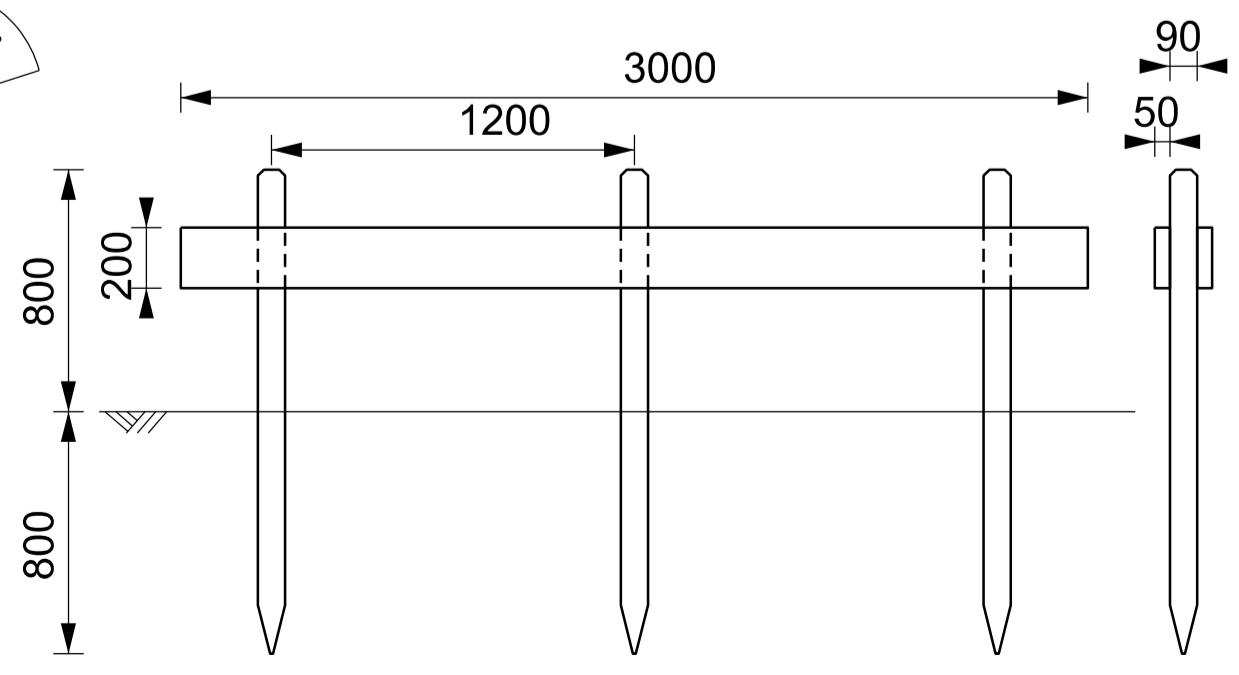
Detail fietsparkeren
